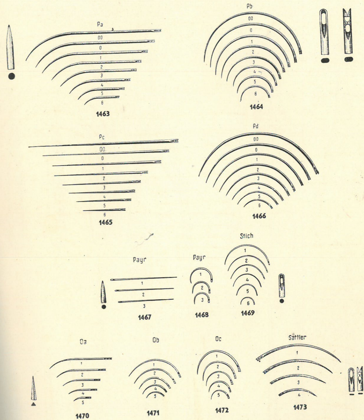
1469 Ace Stich curbe, cu vîrf rotund (fig. 1-6) Aceste ace se produc numai cu urechi obișnuite Ace pentru oftalmologie: Oa, Ob, Oc și model Sattler 1470 Ace Oa cu vîrf triunghiular (fig. 1-5) 1471 Ace Ob cu vîrf triunghiular (fig. 1-5) 1472 Ace Oc cu vîrf triunghiular (fig. 1-5) 1473 Ace Sattler cu vîrf triunghiular (fig. 1-4) Aceste ace se produc cu ambele tipuri de urechi: obișnuite și cu arc
